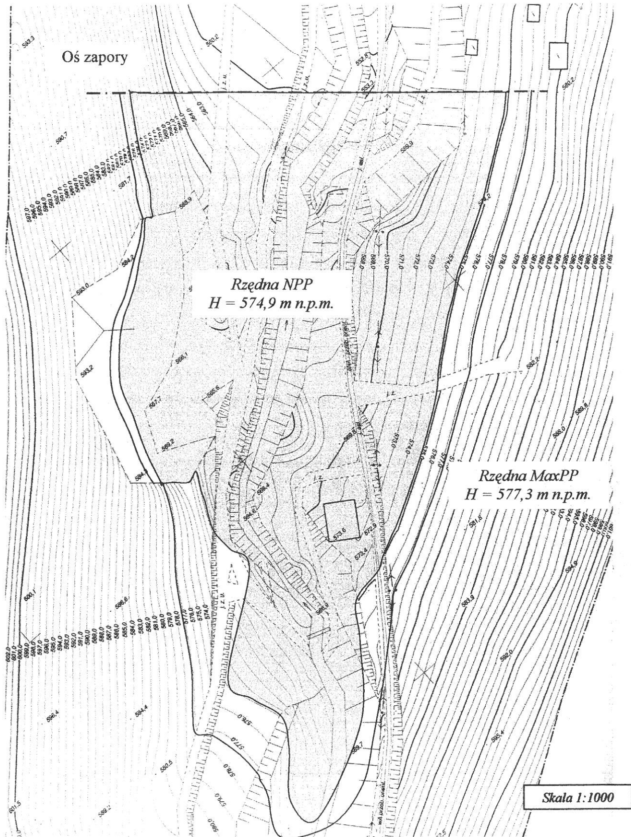
Rys. 7.4. Mapa sytuacyjna zbiornika retencyjnego Bystra na potoku Biała
